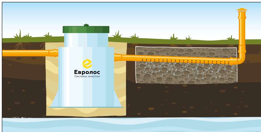
Вариант 6: Монтаж с отводом очищенной воды в фильтрационную траншею неглубокого/поверхностного заложения. Подходит для глины/суглинка.
